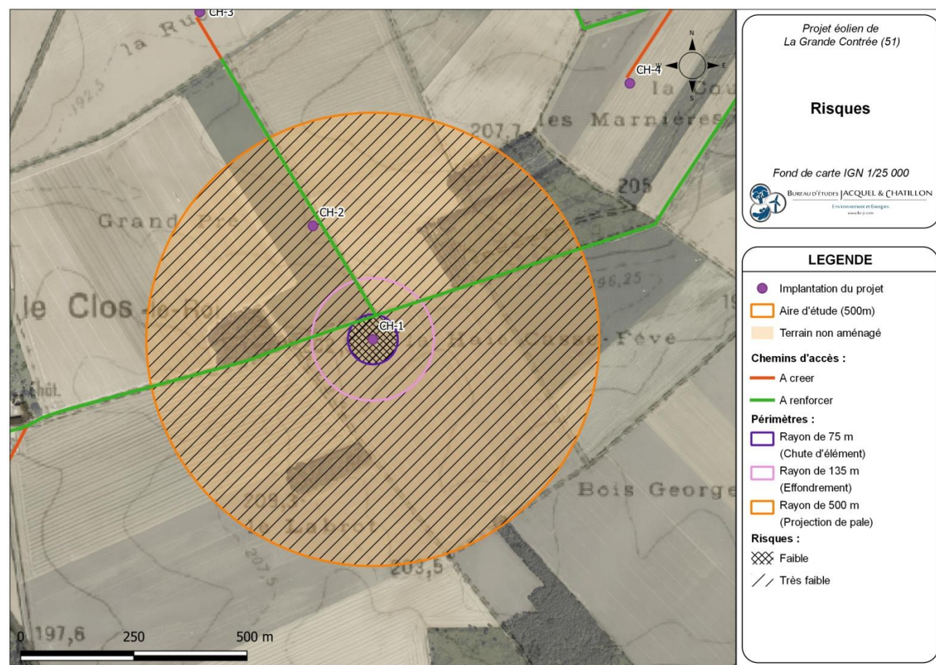
Carte 24 : Éolienne CH-1 – Risques liés à l'effondrement de l'éolienne, à la chute d'élément de l'éolienne, et à la projection de pale ou de fragment de pale (Source : BE Jacquel et Chatillon)
