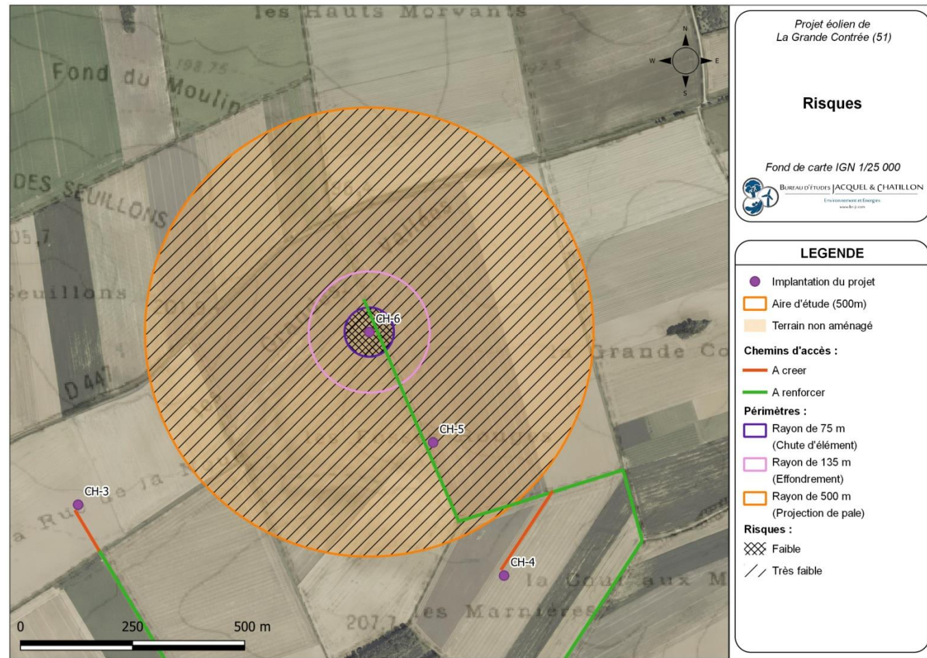
Carte 34 : Éolienne CH-6 – Risques liés à l'effondrement de l'éolienne, à la chute d'élément de l'éolienne, et à la projection de pale ou de fragment de pale (Source : BE Jacquel et Chatillon)
