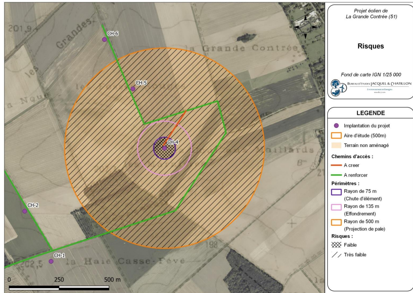
Carte 30 : Éolienne CH-4 – Risques liés à l'effondrement de l'éolienne, à la chute d'élément de l'éolienne, et à la projection de pale ou de fragment de pale (Source : BE Jacquel et Chatillon)
