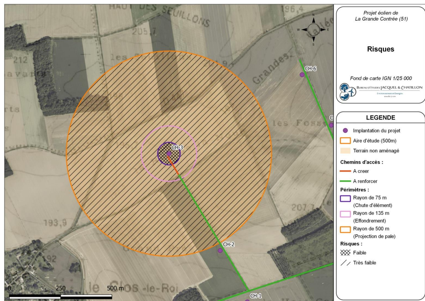
Carte 28 : Éolienne CH-3 – Risques liés à l'effondrement de l'éolienne, à la chute d'élément de l'éolienne, et à la projection de pale ou de fragment de pale (Source : BE Jacquiel et Chatillon)
