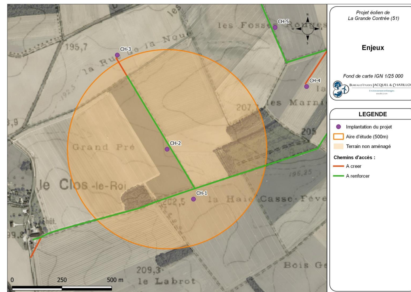
Carte 17 : Éolienne CH-2 – Zones à enjeux (Source : BE Jacquel et Chatillon)
