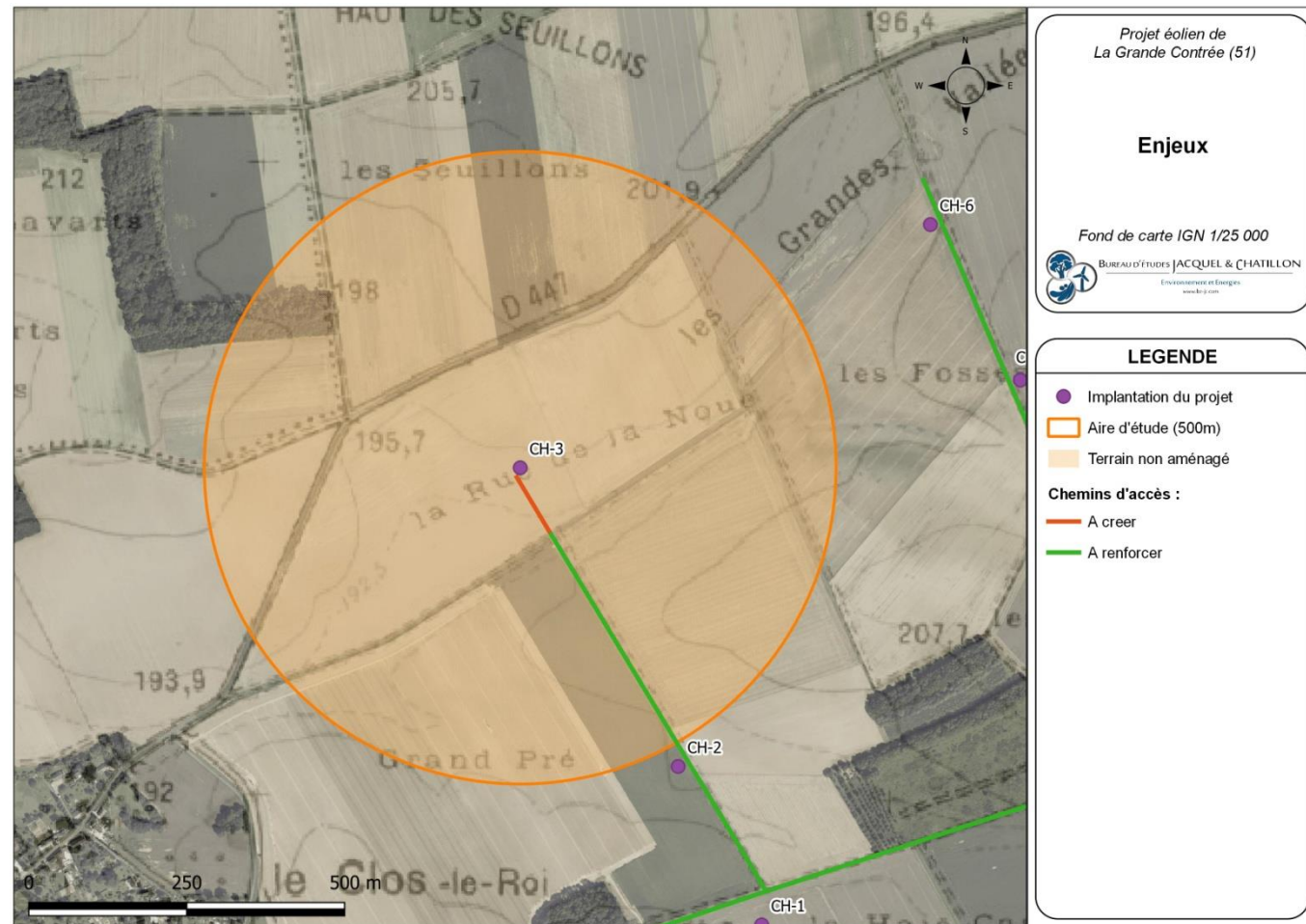
Carte 18 : Éolienne CH-3 – Zones à enjeux (Source : BE Jacquel et Chatillon)
