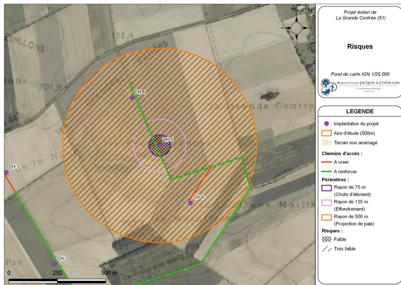
Carte 32 : Éolienne CH-5 – Risques liés à l'effondrement de l'éolienne, à la chute d'élément de l'éolienne, et à la projection de pale ou de fragment de pale (Source : BE Jacquiel et Chatillon)
