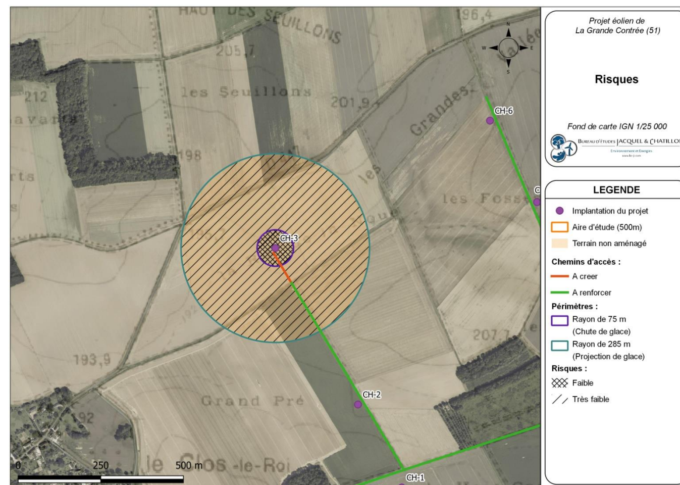
Carte 29 : Éolienne CH-3 – Risques liés à la chute et à la projection de glace (Source : BE Jacquiel et Chatillon)
