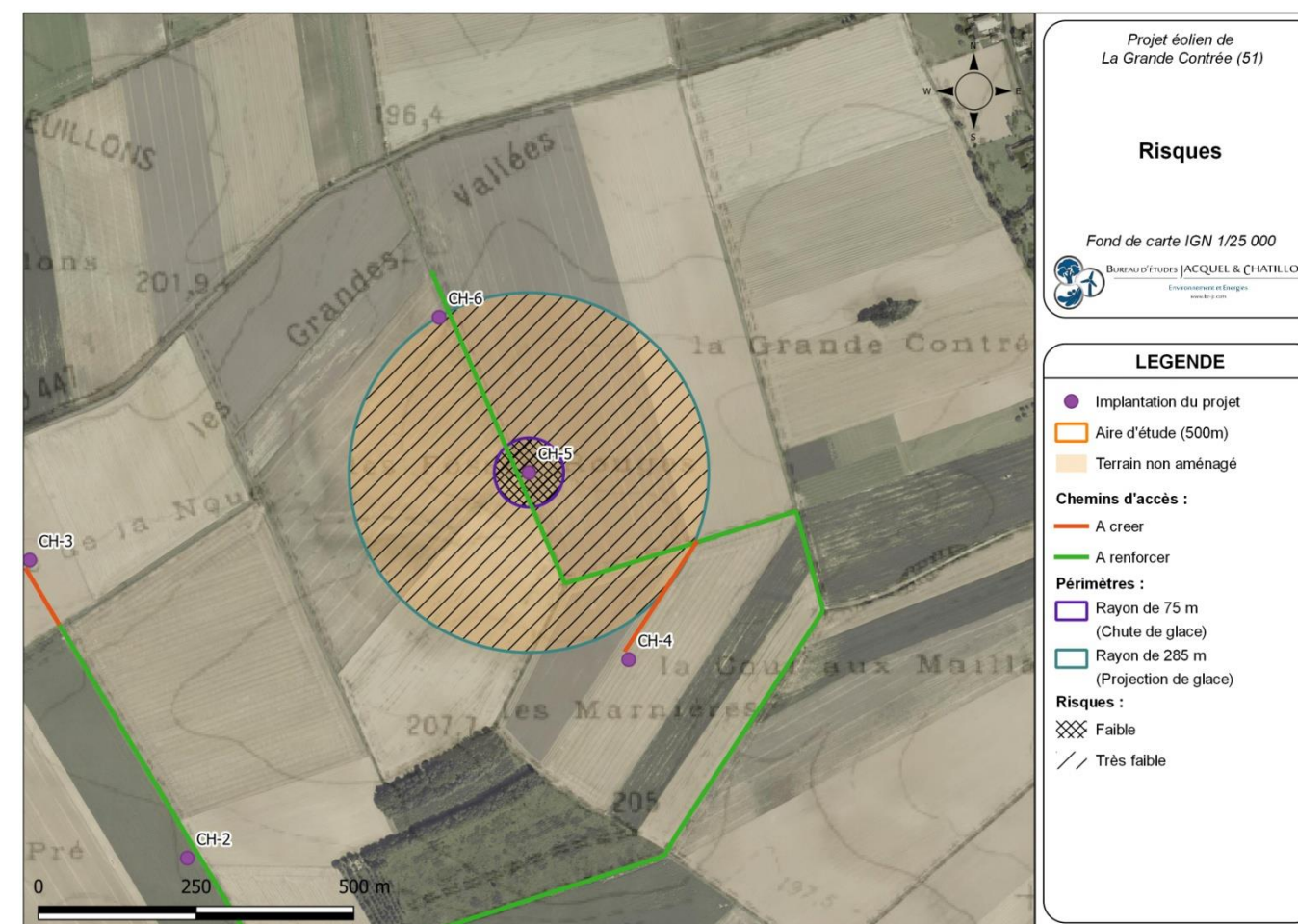
Carte 33 : Éolienne CH-5 – Risques liés à la chute et à la projection de glace (Source : BE Jacquiel et Chatillon)
