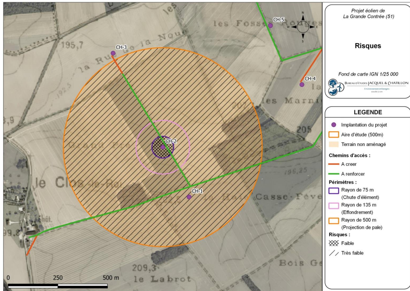
Carte 26 : Éolienne CH-2 – Risques liés à l'effondrement de l'éolienne, à la chute d'élément de l'éolienne, et à la projection de pale ou de fragment de pale (Source : BE Jacquel et Chatillon)
