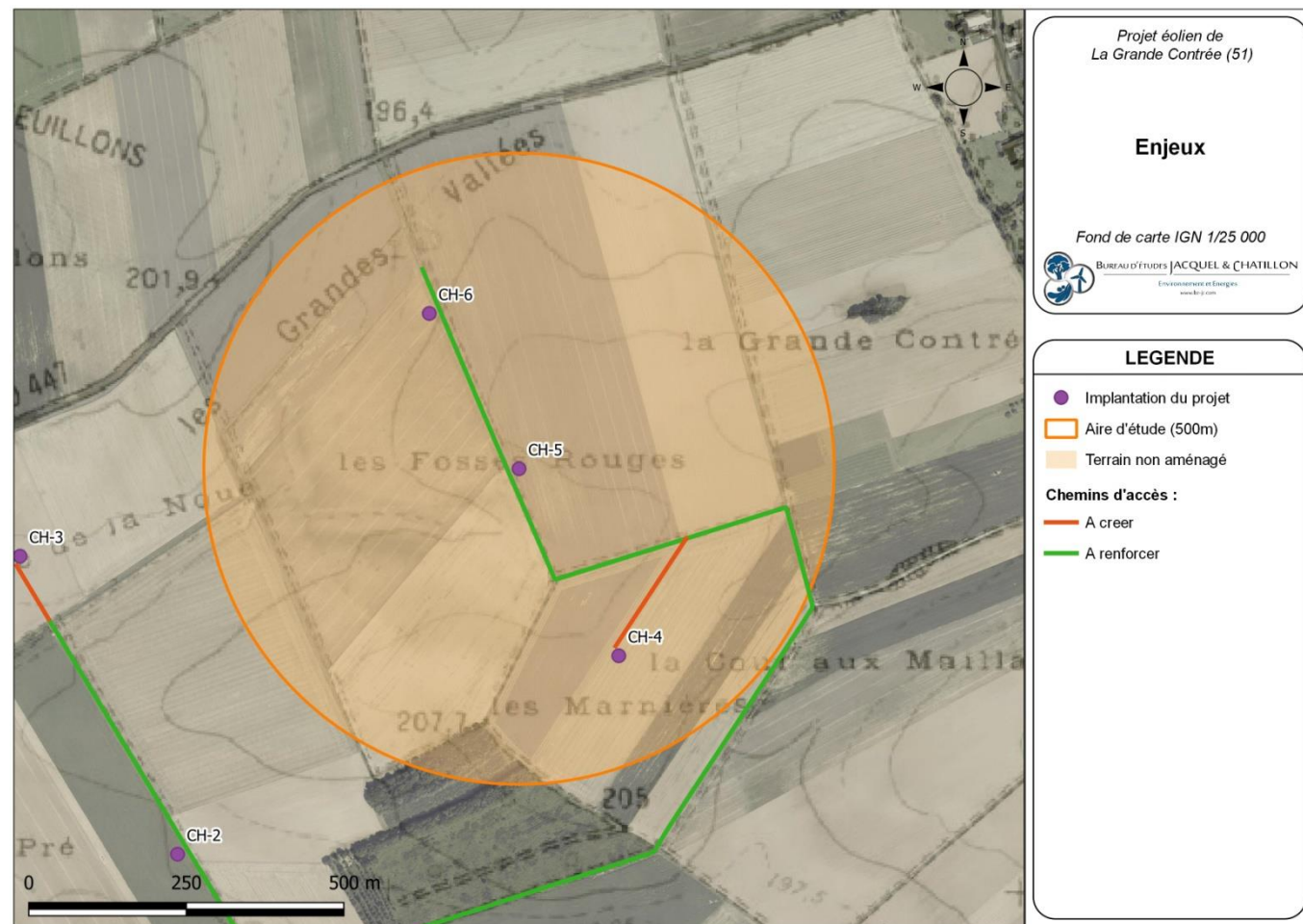
Carte 20 : Éolienne CH-5 – Zones à enjeux (Source : BE Jacquel et Chatillon)
