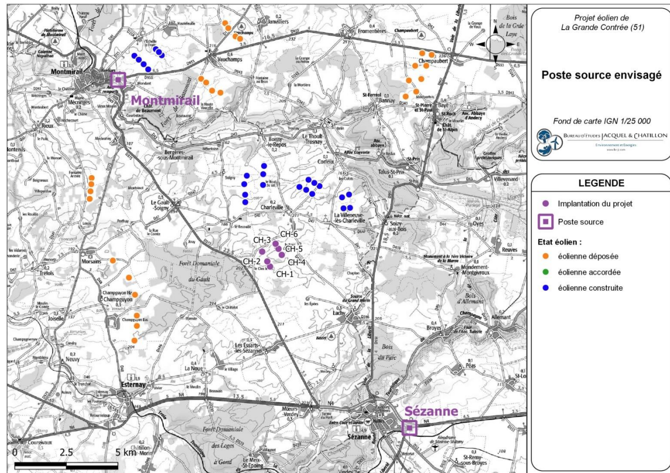
Carte 23 : Hypothèses pour le raccordement au poste-source (Source : BE Jacquel et Chatillon)
