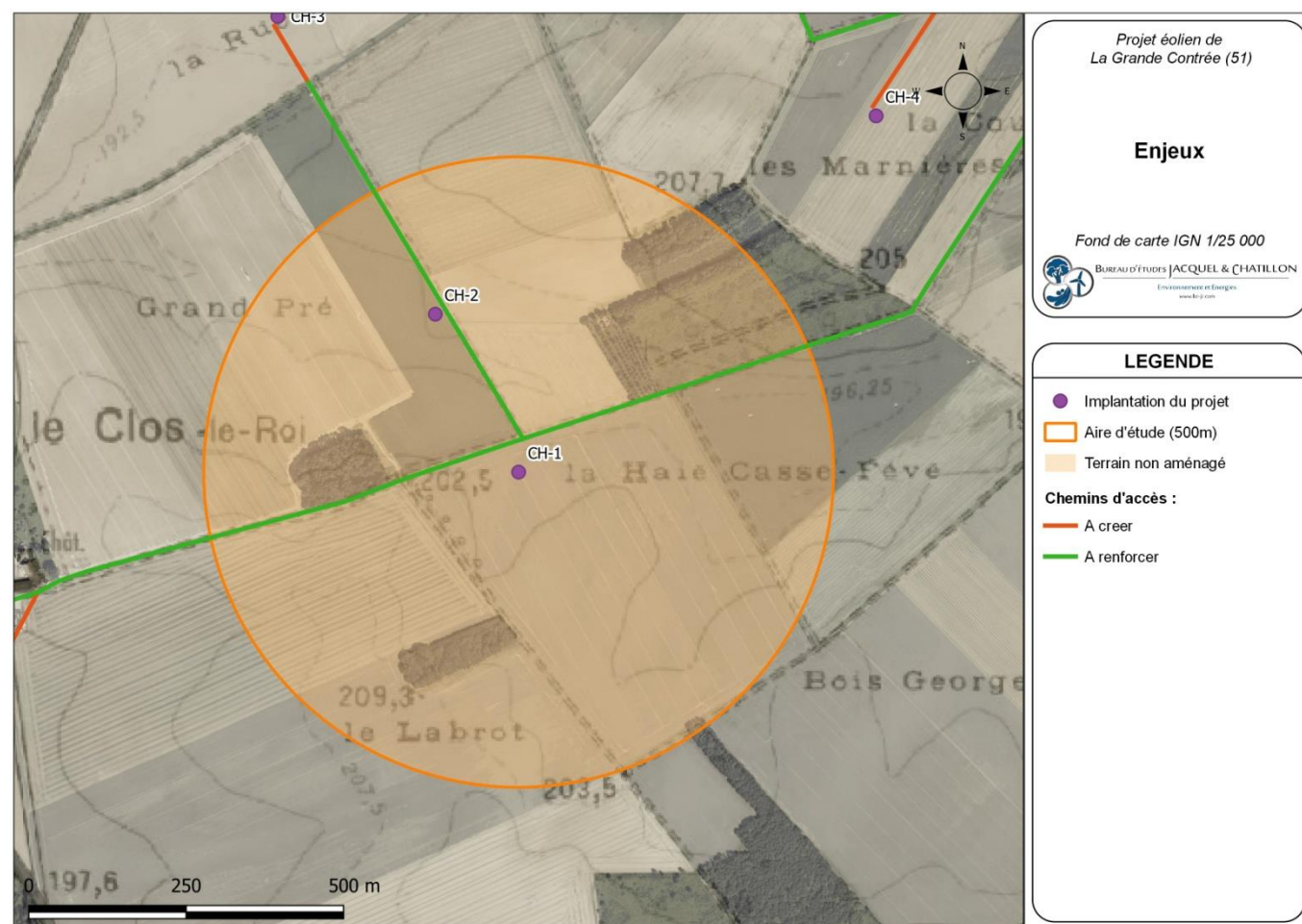
Carte 16 : Éolienne CH-1 – Zones à enjeux (Source : BE Jacquel et Chatillon)
